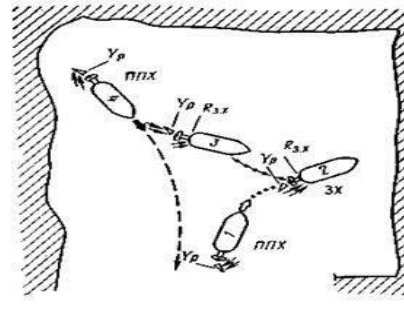
Рис. 14.9. Маневрирование судна на ограниченной акватории: ППХ — полный передний ход; ЗХ — задний ход
